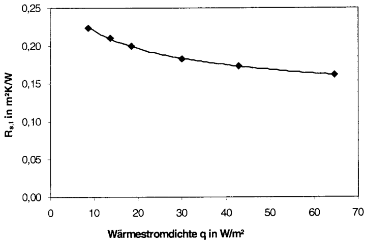
Bild 2 Gesamtwärmeübergangswiderstand
