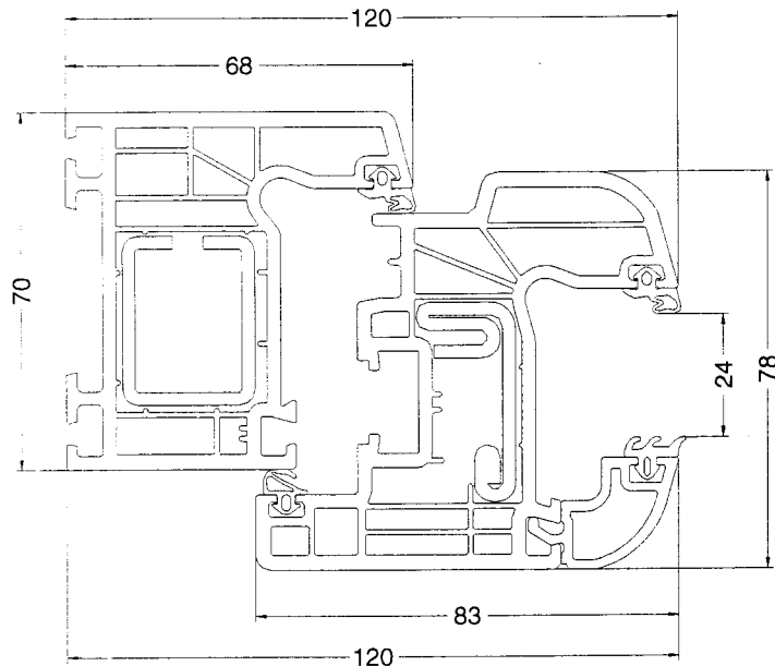
Bild 1 Zeichnung Querschnitt
