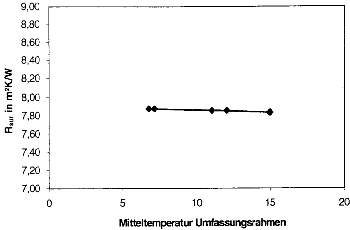
Bild 1 Wärmedurchlasswiderstand Umfassungsrahmen
